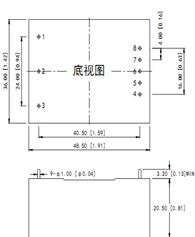
塑料壳尺寸
