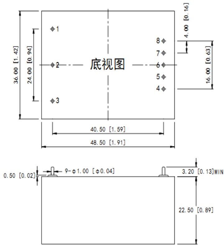
金属壳尺寸
