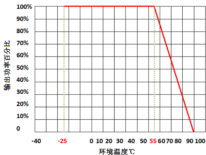
温度曲线图
