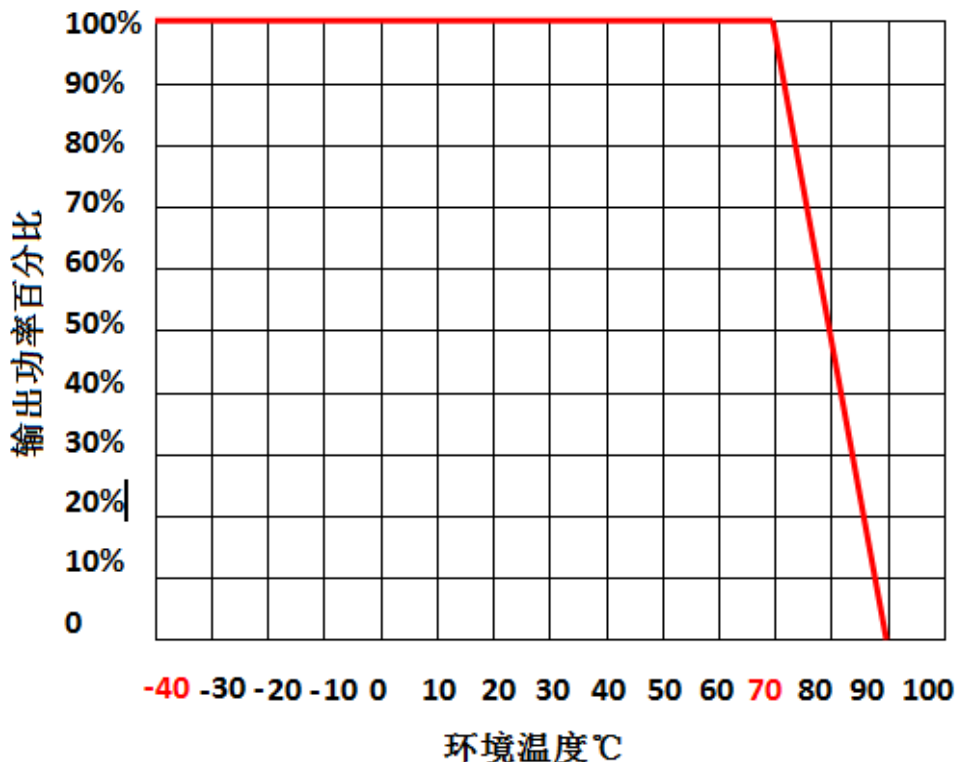
温度曲线图
